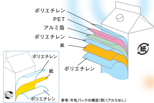
参考:牛乳パックの構造(例)(アルミなし)
